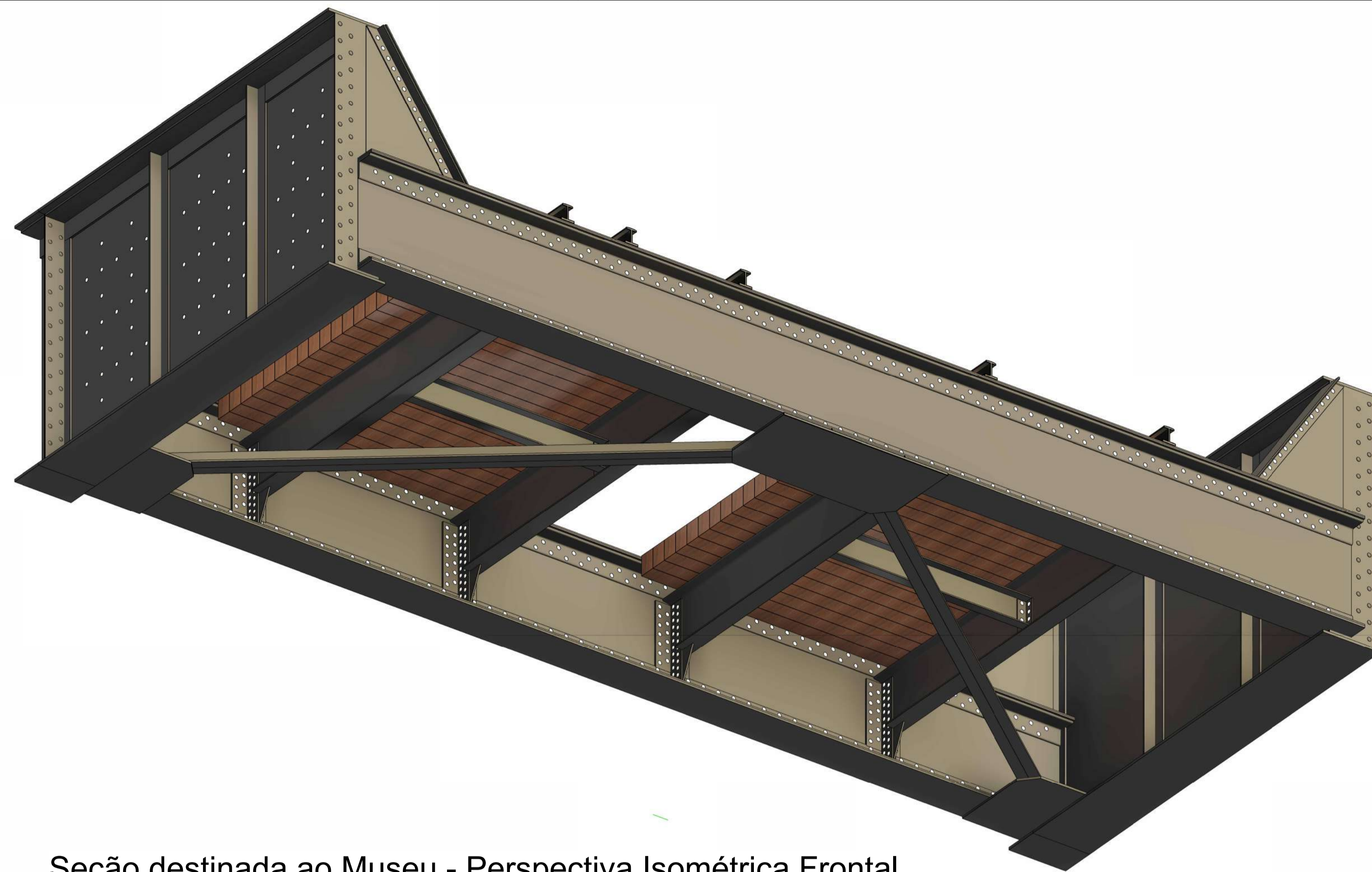
Seção destinada ao Museu - Perspectiva Isométrica Frontal Inferior Esc.: 1/25
