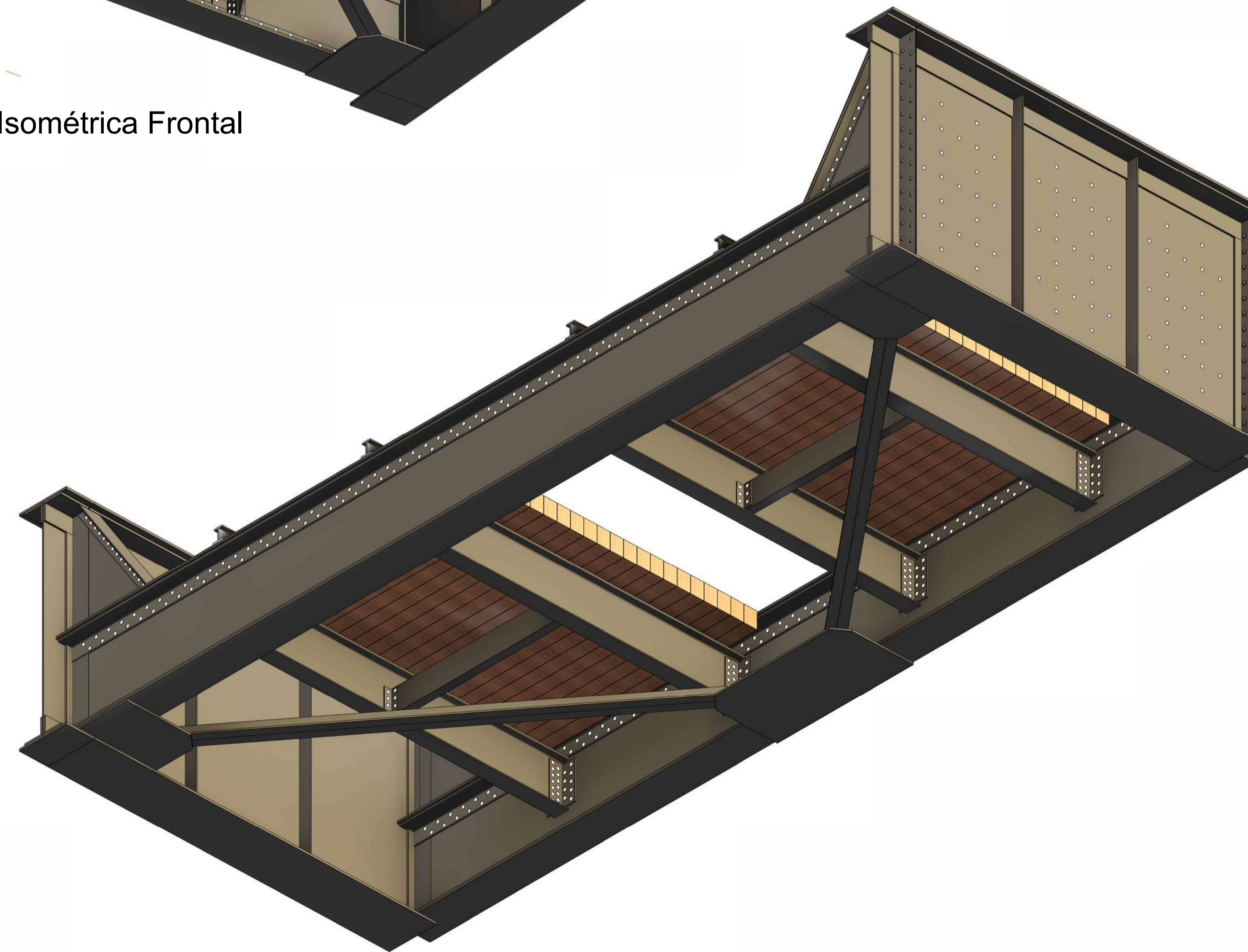
Seção destinada ao Museu - Perspectiva Isométrica Posterior Inferior Esc.: 1/25
