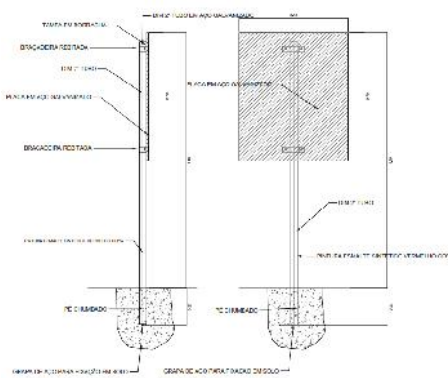
Imagem 3: Especificações técnicas do suporte
